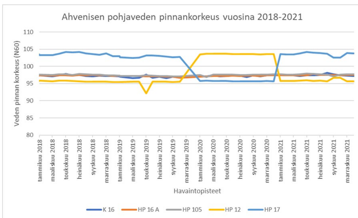
Kuva 3 Ahvenisen pohjaveden korkeus vuosina 2018–2021. Korjaus 12.12.2022: HP 12 ja HP 17 -putkien tulokset ovat sekoittuneet vuoden 2020 osalta.
